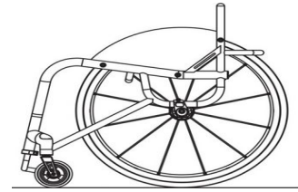
XA080 - Estrutura fechada
