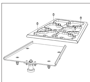
MC 41 Adaptação trapezoidal para órteses de assento
